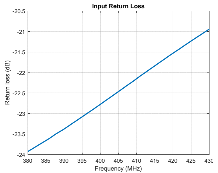
نتایج اندازه‌گیری افت بازگشتی ماژول UHF
