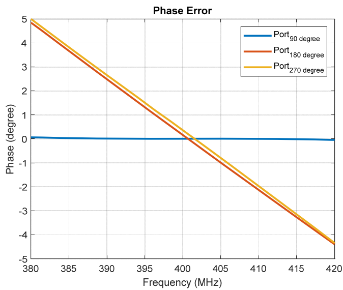
نتایج اندازه‌گیری خطای فاز پورتهای ماژول UHF نسبت به پورت ۲ با در نظر گرفتن فاز صفر درجه برای آن
