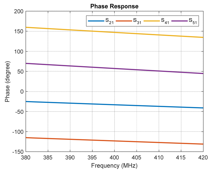
نتایج اندازه‌گیری پاسخ فاز پورتهای ماژول UHF
