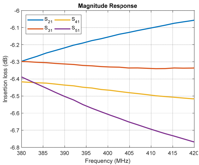
نتایج اندازه‌گیری پاسخ دامنه پورتهای ماژول UHF
